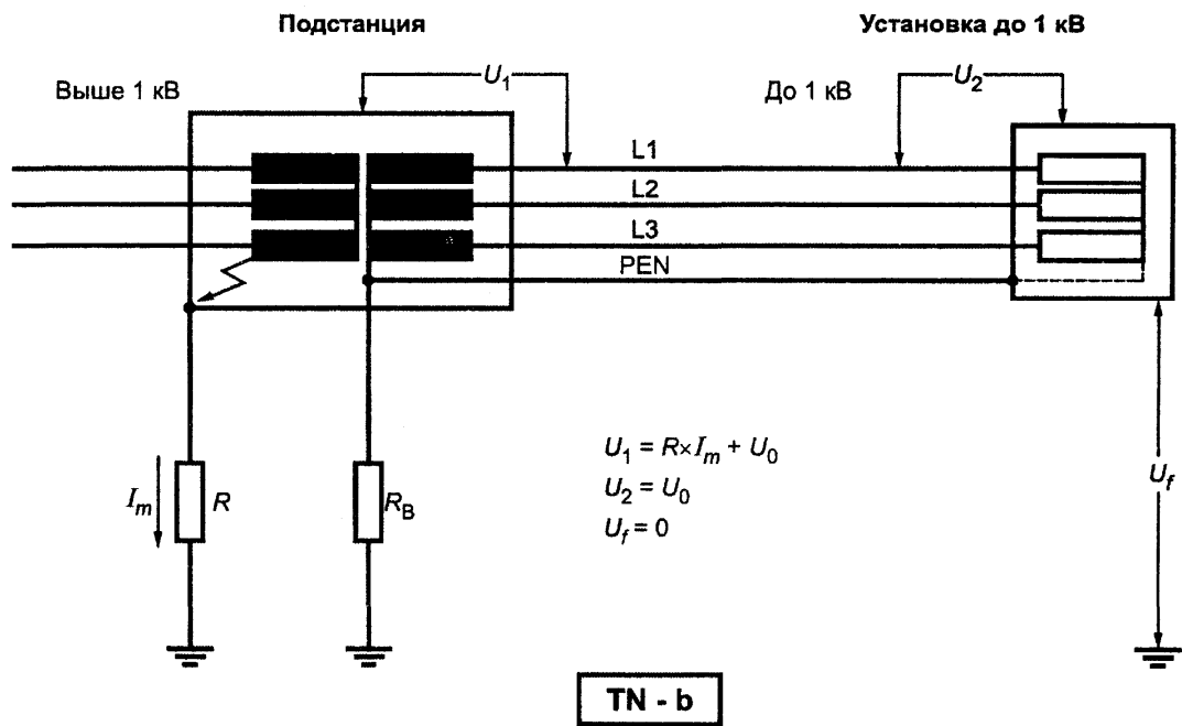
Рисунок 44В — TN-системы
