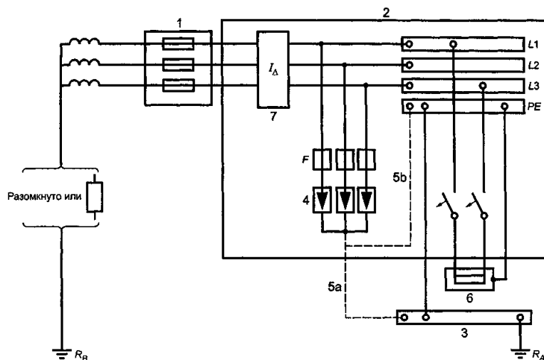
1 — ввод распределительной сети; 2 — распределительный щит; 3 — главный заземляющий зажим (шина); 4 — УЗИП; 5а, 5b — заземление УЗИП; 6 — защищаемое оборудование; 7 — УДТ; F — защитное устройство, указанное изготовителем (предохранитель, автоматический выключатель, УДП); R_A — заземляющий электрод (сопротивление); R_B — заземляющий электрод (сопротивление) системы питания
